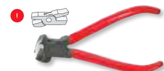
Nr. 1111 STUBAI Vorschneider N° 1111 STUBAI End cutting nippers
