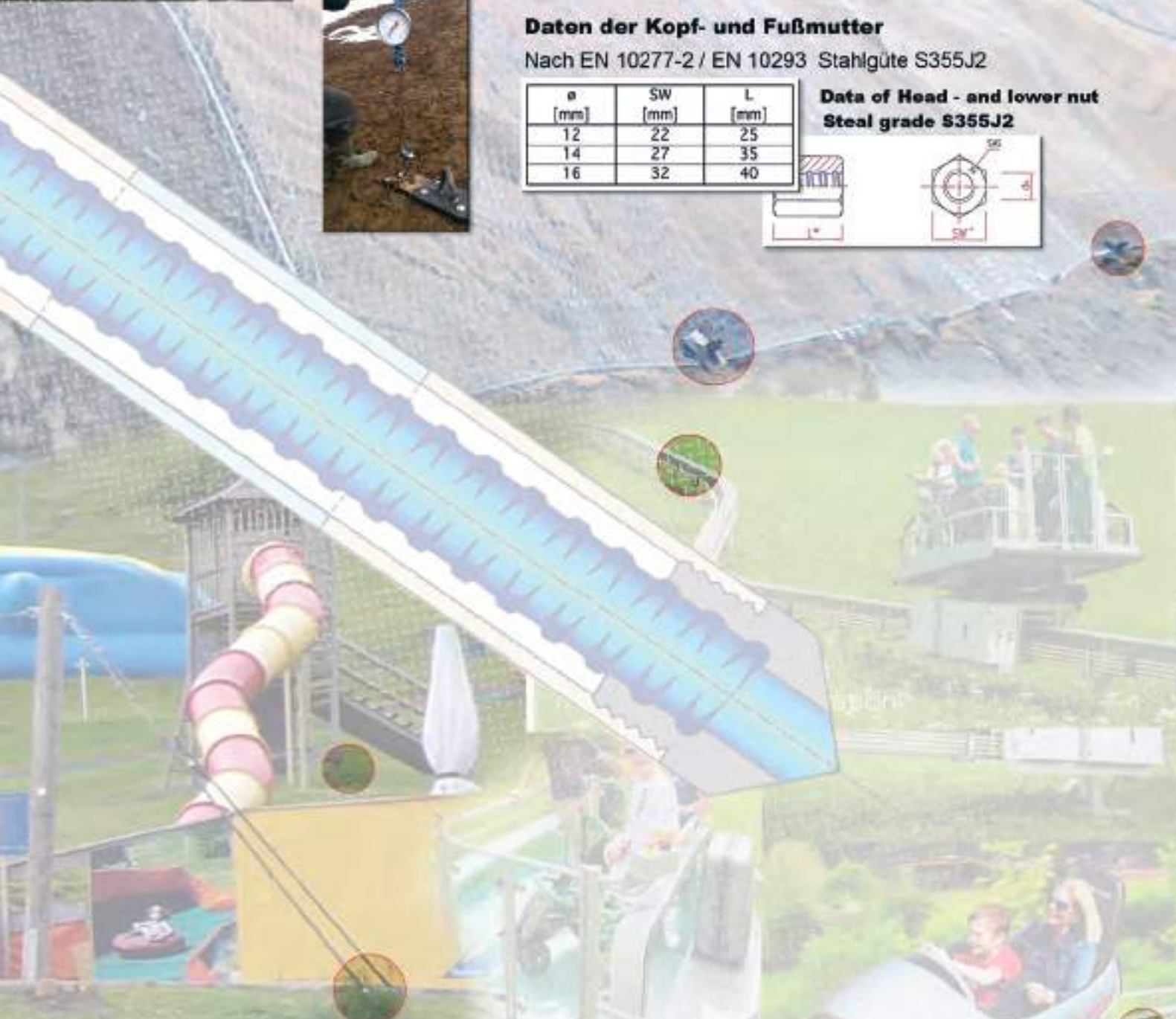
Abbildung 1: Seilbefestigung nach dem Bauwerk
