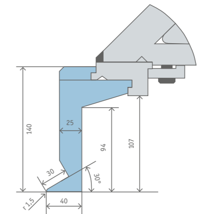
GEISSFUSSSCHIENE KLICKSYSTEM 107 MM, HINTEN FREI
