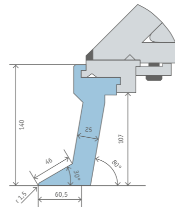
GEISSFUSSSCHIENE KLICKSYSTEM 107 MM, VORNE FREI
