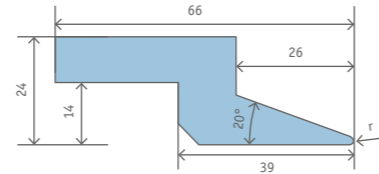
SCHARFSCHIENE 66/24 20° GEKRÖPFT
