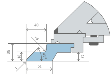
SCHARFSCHIENE 45° R=2 MIT KLICKSYSTEM
