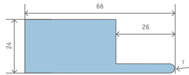
RUNDSCHIENE 66/24 R = 1,5 - 12
