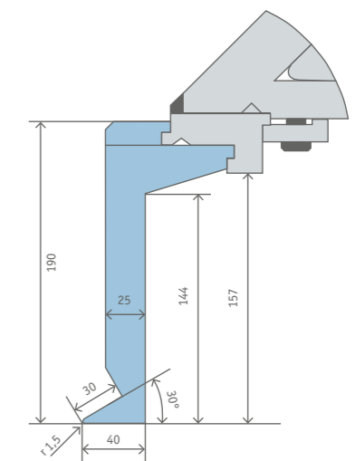
GEISSFUSSSCHIENE KLICKSYSTEM 157 MM, HINTEN FREI
