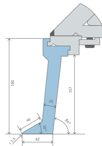
GEISSFUSSSCHIENE KLICKSYSTEM 157 MM, VORNE FREI
