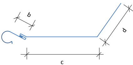
Variante B: Flach mit Aufkantung
