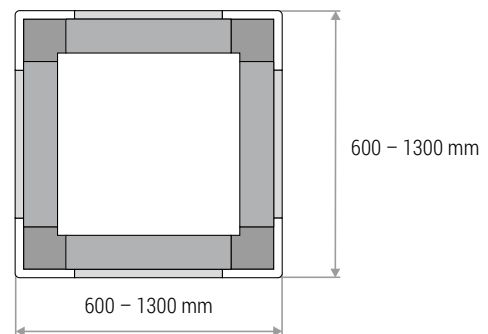
Kaminkranz VARIO, Maßbereich
