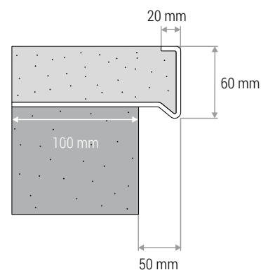
Umlaufender Überstand 50 mm
