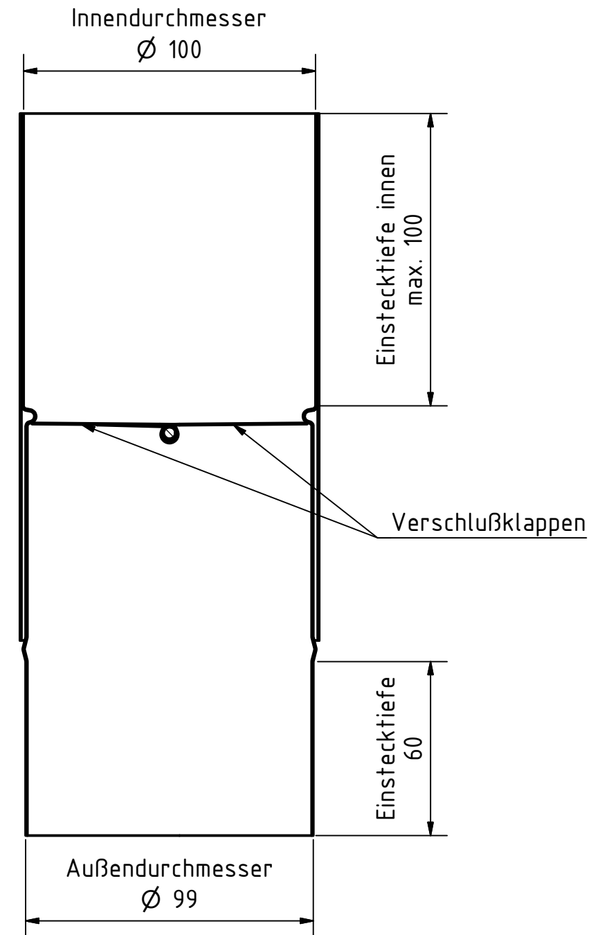
Schnitt A-A
