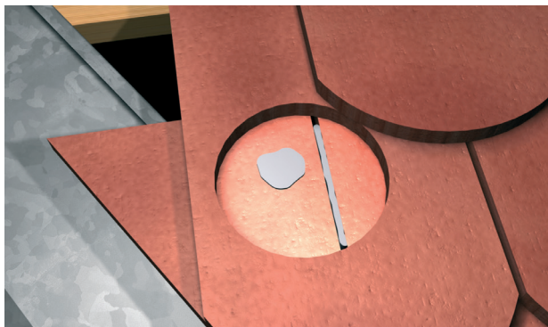
Anwendungsbeispiel: Montageverklebung von Zuschnitten bei Dachsteinen und -ziegeln
