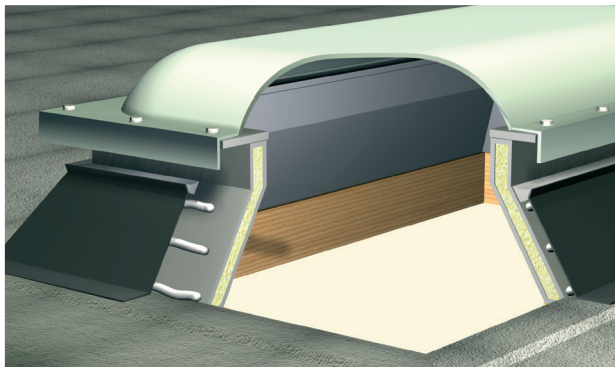
Anwendungsbeispiel: WOLFIN-Verbundbleche beim Lichtkuppelanschluss
