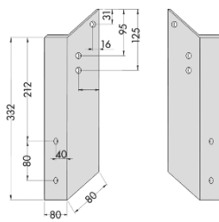
Dachsparrenhalter
