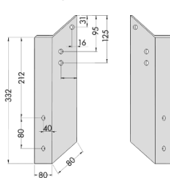
Dachsparrenhalter
