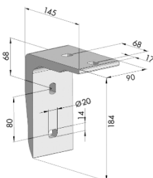
Deckenhalter
