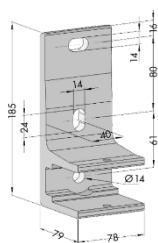
Wandhalter
