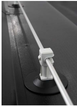
Einsatz von Blitzableiter- stützen auf z.B. Attikakronen
