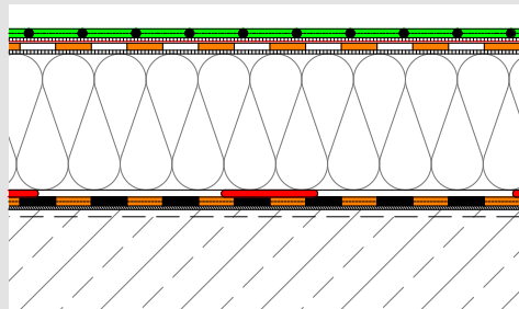
Geklebter Schichtenaufbau
